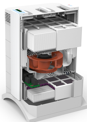
sezione
